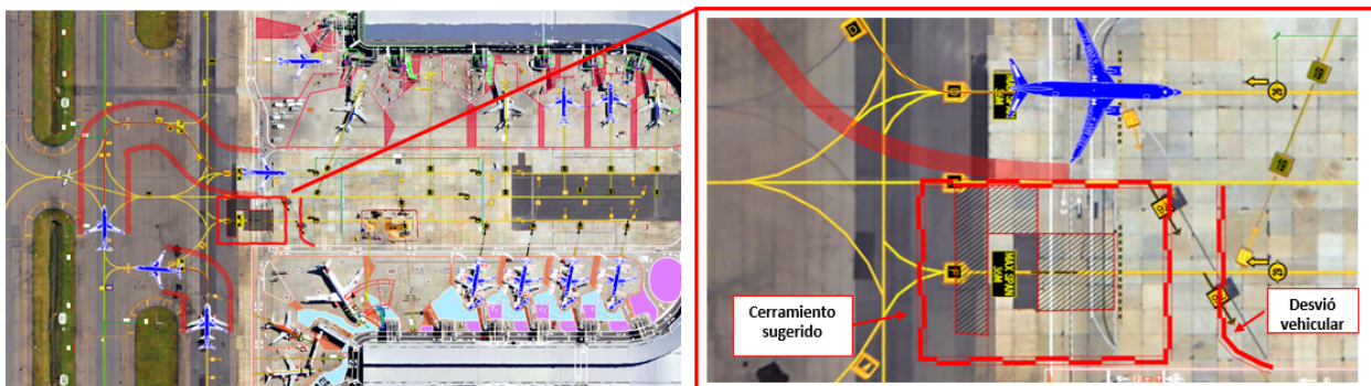
Figura 1: desvío vehicular calle de servicio externa plataforma central entre PSN 76 y TWY F-E
